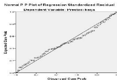
GAMBAR 4.2 HASIL UJI NORMALITAS MENGGUNAKAN PROBABIL
