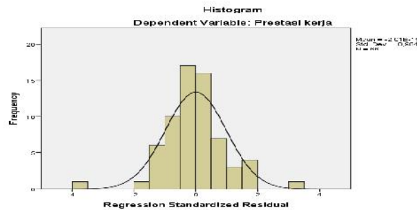
GAMBAR 4.1 HASIL UJI NORMALITAS MENGGUNAKAN HISTOGRAM
