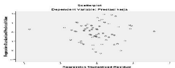
GAMBAR 4.3 HASIL UJI NORMALITAS MENGGUNAKAN SCATTERPLOT
