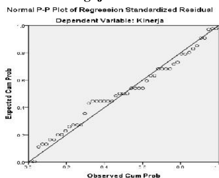
Gambar 4.10 Hasil Pengujian Normalitas
