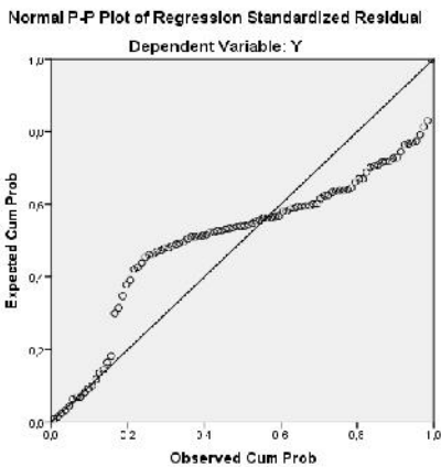
Gambar 4.1 Uji Normalitas
